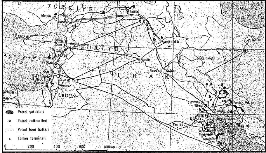
Şekil 5- Basra Körfezi-Akdeniz Arasındaki Petrol Boru Hatları Figure 5- Oil Pipelines Between the Persian Gulf and the Mediterranean
